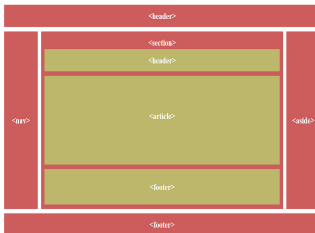
EstructuraWebBasica.html
